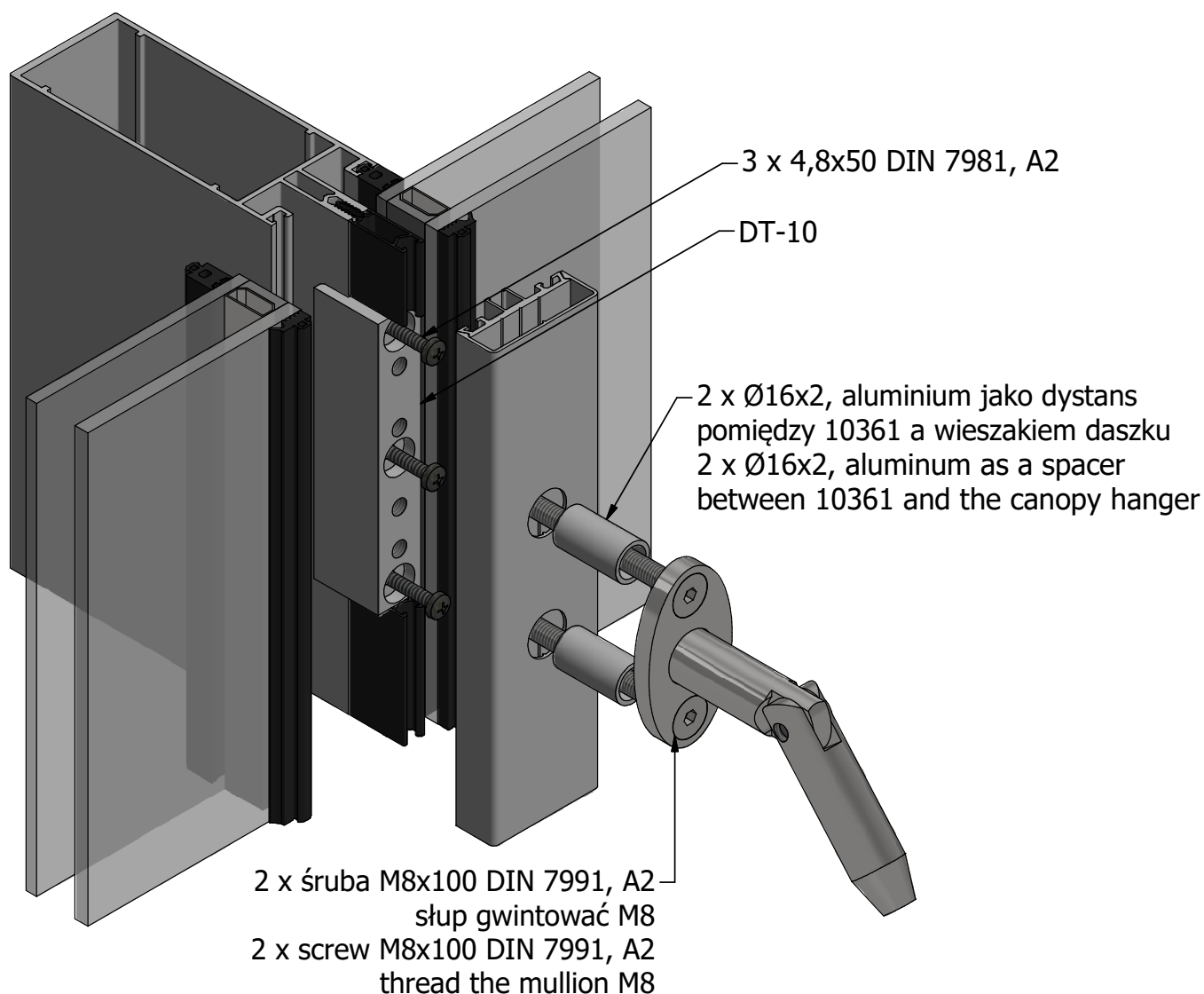
Kostka mocująca do daszków całoszklanych i lameli Fixing block for all-glass canopies and lamellae
