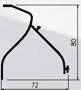
Lamela 70V górna - obwód: 388mm - długości handlowe: 6000mm - surowa, nr. esco: 56-721484 - RAL, nr. esco: 56-721492
