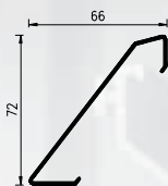
Lamela 75 L - długości handlowe: 6000mm - surowa, nr. esco: 56-885061 - RAL, nr. esco: 56-885070
