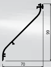
Lamela 70S - obwód: 321mm - długości handlowe: 6000mm - surowa, nr. esco: 56-651770 - RAL, nr. esco: 56-721441
