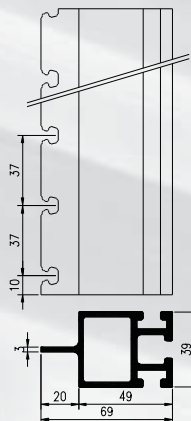
Profil-Uchwył 40/70 do 30Z & 50Z - długości handlowe: 6000mm - surowa, nr. esco: 56-884790 - RAL, nr. esco: 56-884804
