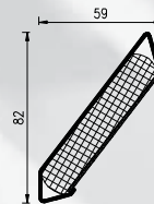
Lamela akustyczna 75 Z - długości handlowe: 6000mm - RAL, nr. esco: 56-885088
