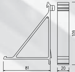
Klips 90S & 90HP – czarny, nr. esco: 56-689939
