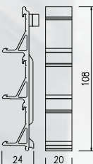
Klips 20Z – 35V/3 – czarny, nr. esco: 56-650544
