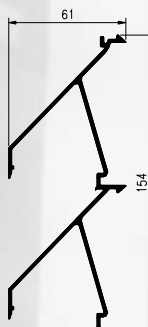
Podwójna lamela 50Z NP
