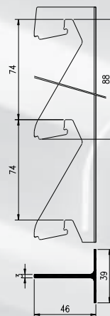
Klips 40/47 - profil długość 6000mm - surowy, nr. esco: 56-721611 - RAL, nr. esco: 56-721620
