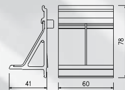
Klips 50 / 75 & 80HP łączący – czarny, nr. esco: 56-652334
