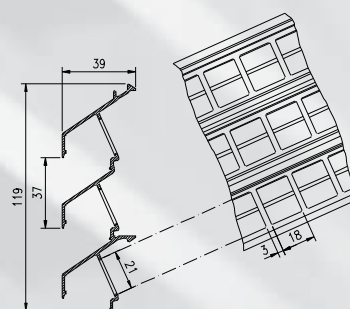
Potrójna lamela 30Z P2
