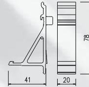
Klips 50 / 75 & 80HP – czarny, nr. esco: 56-651133
