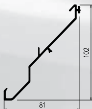
Lamela 80HP - obwód: 361mm - długości handlowe: 6000mm - surowa, nr. esco: 56-721506 - RAL, nr. esco: 56-721514
