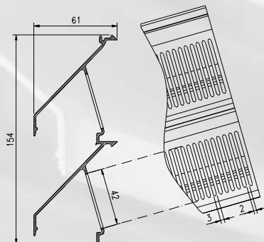
Podwójna lamela 50Z P1
