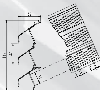
Potrójna lamela 30Z P1
