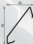
Lamela 75 Z - długości handlowe: 6000mm - surowa, nr. esco: 56-885061 - RAL, nr. esco: 56-885070
