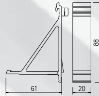
Klips 70S – czarny, nr. esco: 56-651788
