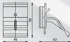
Klips 75 L/Z - łączący - nr. esco: 56-885100
