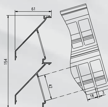
Podwójna lamela 50Z P2
