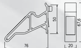
Klips 60C – czarny, nr. esco: 56-721590
