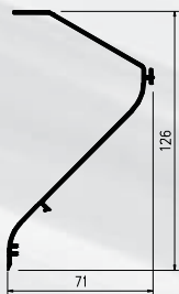
Lamela 70S górna - obwód: 433mm - długości handlowe: 6000mm - surowa, nr. esco: 56-721450 - RAL, nr. esco: 56-721468
