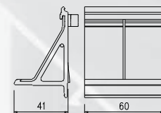
Klips 50S / 50Z / 70V łączący – czarny, nr. esco: 56-650641
