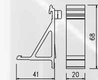
Klips 50S / 50Z / 70V – czarny, nr. esco: 56-650552
