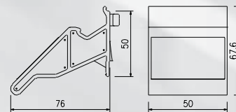
Klips 60C łączący – czarny, nr. esco: 56-733717
