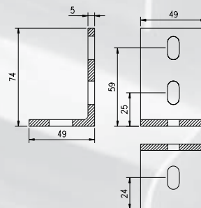
Łapa montażowa L75x50x5 - długości handlowe: 6000mm - surowa, nr. esco: 56-651125 - RAL, nr. esco: 56-775711
