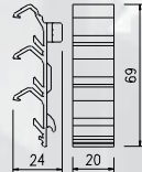
Klips 20V/3 – czarny, nr. esco: 56-651192
