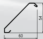
Lamela 60C - obwód: 217mm - długości handlowe: 6000mm - surowa, nr. esco: 56-721522 - RAL, nr. esco: 56-721530
