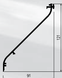
Lamela 90S - obwód: 379mm - długości handlowe: 6000mm - surowa, nr. esco: 56-689890 - RAL, nr. esco: 56-721850
