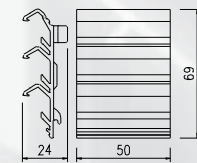
Klips 20V/3 łączący – czarny, nr. esco: 56-721581
