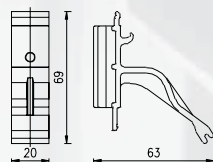
Klips 75 L/Z - nr. esco: 56-885096
