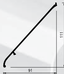
Lamela 70S górna - obwód: 433mm - długości handlowe: 6000mm - surowa, nr. esco: 56-721450 - RAL, nr. esco: 56-721468
