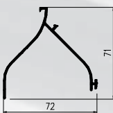
Lamela 70V - obwód: 337mm - długości handlowe: 6000mm - surowa, nr. esco: 56-704466 - RAL, nr. esco: 56-721476
