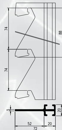
Klips 21/73 - profil długość 6000mm - surowy, nr. esco: 56-884839 - RAL, nr. esco: 56-884847
